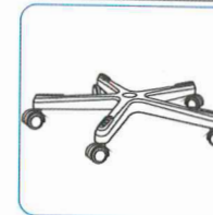
6 Montați roțile
